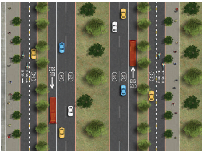
Figura 43. Ejemplos de solución para avenidas con laterales.
