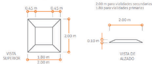
Figura 33. Dimensiones y efecto de los cojines. Fuente: (ITDP/I-CE, 2011)
