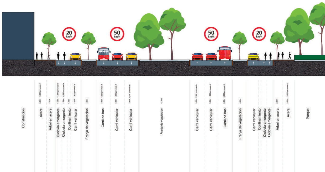
Figura 4. Configuración estándar de una vía primaria
