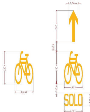
Figura 23. Identificación de vía ciclista exclusiva. (Fuente: SEMOVI, 2020)
