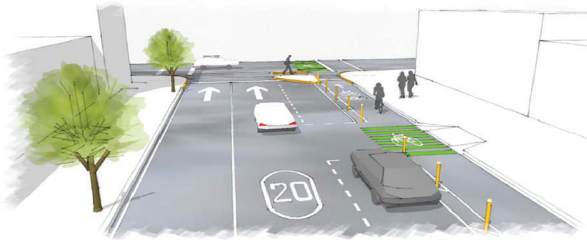
Figura 27. Ciclovía unidireccional confinada por cordón de estacionamiento. (Fuente: CONAPRA, ITDP; 2016)
